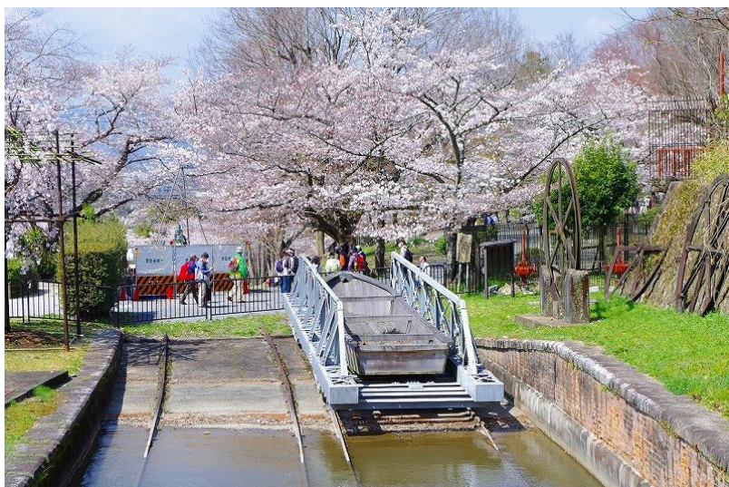
蹴上インクライン／船を台車に乗せて移動するシステム
